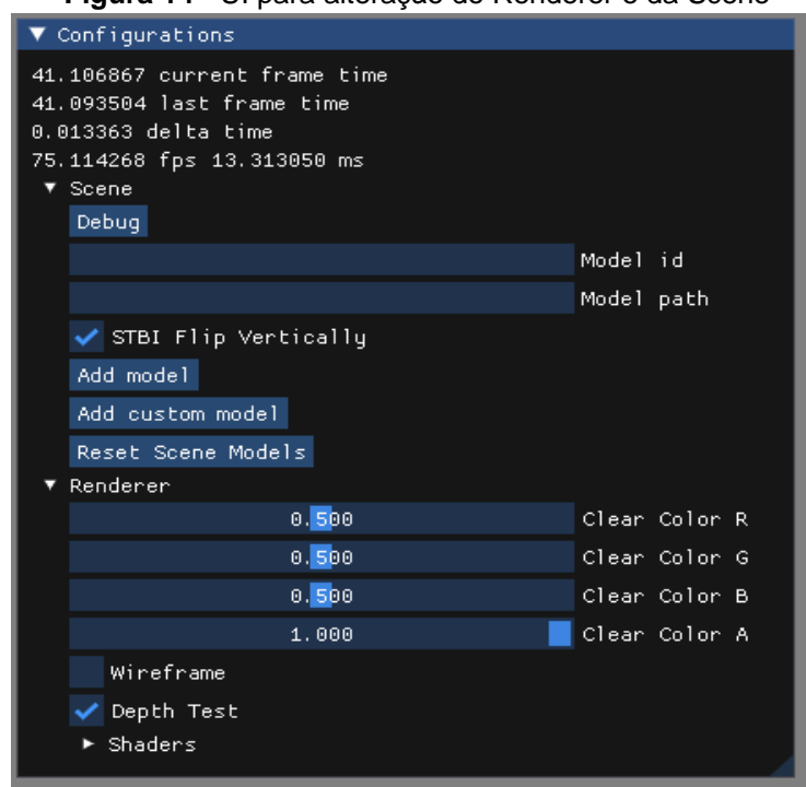
Figura 14 - UI para alteração do Renderer e da Scene
