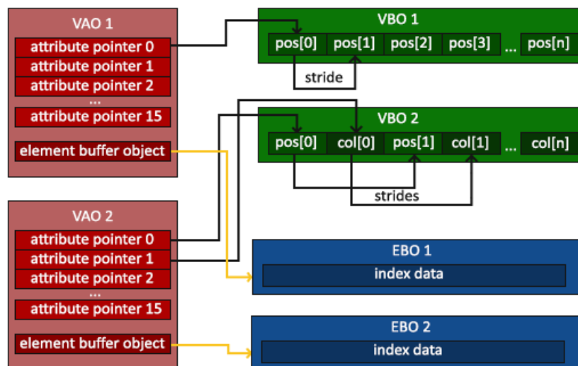
Figura 3 - Funcionamento de VAO, VBO e EBO
